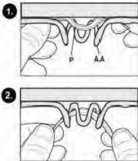
Крепление сетки P на кольцо AA
