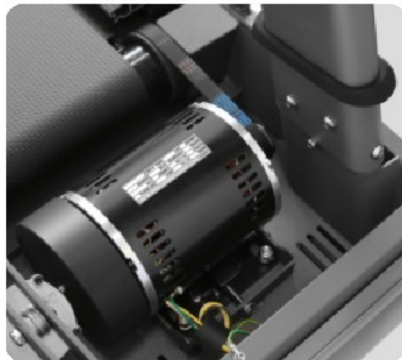
ДВИГАТЕЛЬ LEESON МОЩНОСТЬЮ 3,5 Л.С. (AC)
