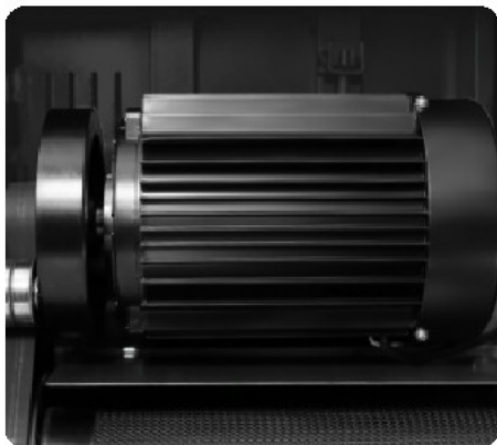
ДВИГАТЕЛЬ LEESON МОЩНОСТЬЮ 4,0 Л.С. (AC)
