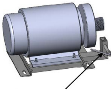
Регулировочный болт
